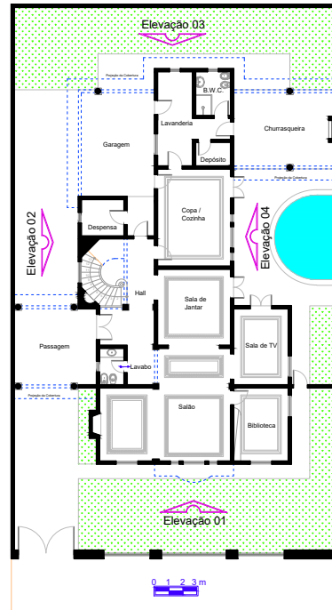
Térreo
