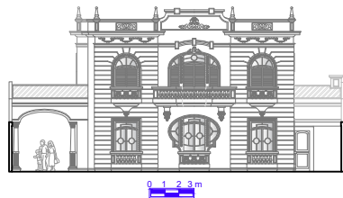
Elevação 01
