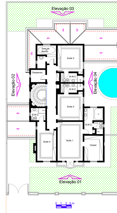
Superior
