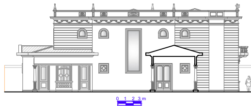
Elevação 02
